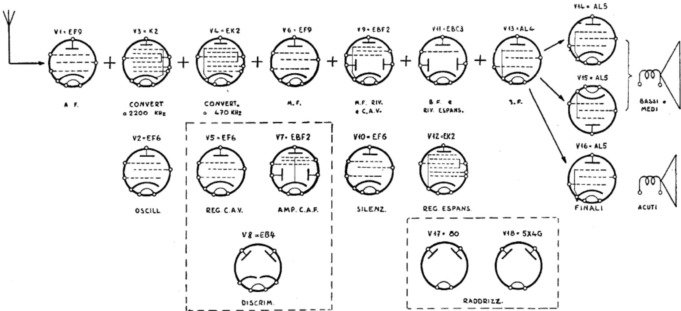
- Utilizzazione delle 18 valvole del ricevitore di cui le figure 137, 138 e 139. (Phonola, mod. 1800/1).
